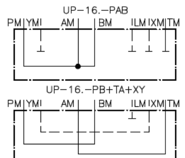
UP-16.-PT UP-16.-PT-XY UP-16.-PAB UP-16.-PA+TB UP-16.-PB+TA UP-16.-PB+TA+XY
