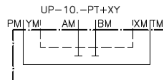
UP-10.-PT+XY UP-10.-PA+TB+XY
