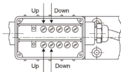
Rampeneinstellung für Slave-Magnet
