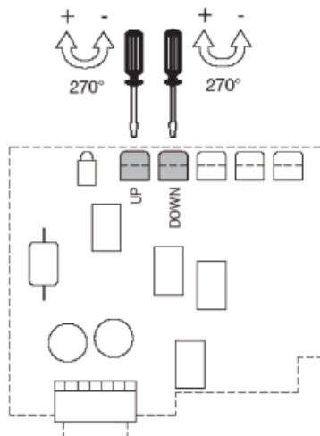
Rampeneinstellung für Master-Magnet
