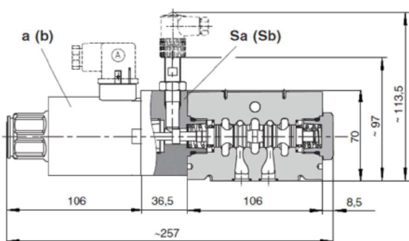
Wegeventile, 2 Schaltstellungen
