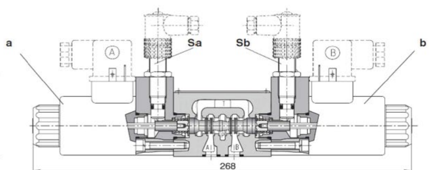
Wegeventile, 3 Schaltstellungen
