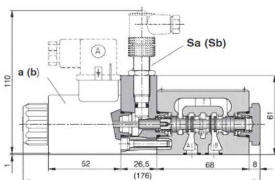
Wegeventile, 2 Schaltstellungen
