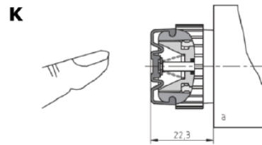
Nothandbetätigung mit Gummischutzhülle
