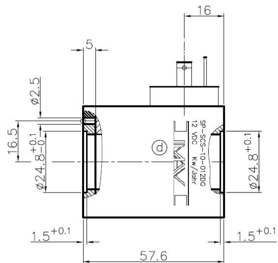
G-Stecker
