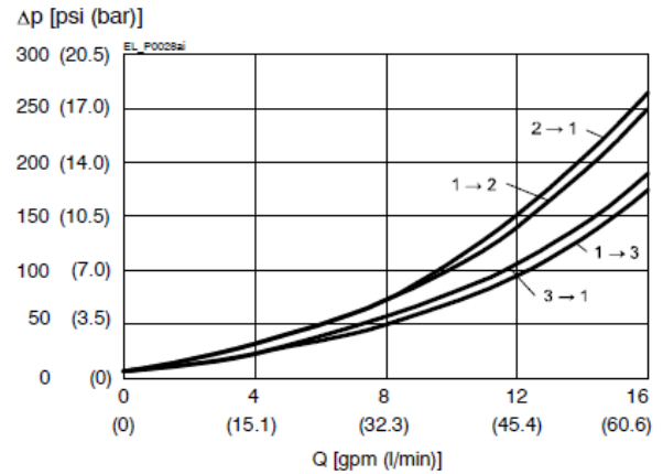
p = f(Q) Druck-Verstellverhalten – ESDV-12-3D
