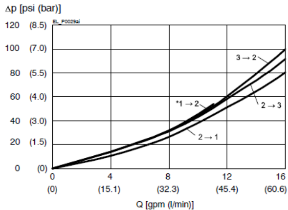
p = f(Q) Druck-Verstellverhalten – ESDV-12-3C
