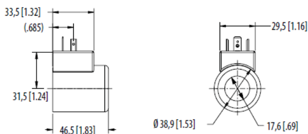
G0 DIN 43650
