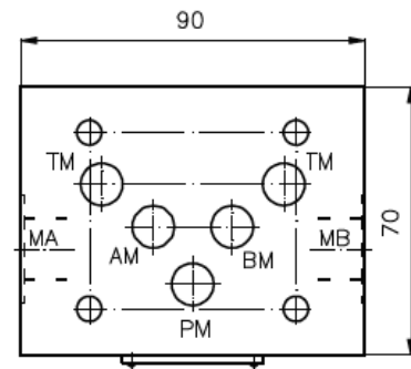
MPZ-10.-A+B-B..
