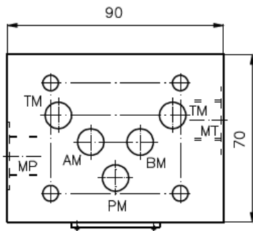
MPZ-10.-P-B.. MPZ-10.-P+T-B..
